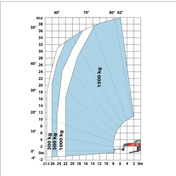
Drehung mit abgelassenen Stützen und 2 to jib (Metrisch) Maschine auf abgesenkten Stabilisatoren mit 1500 kg Winde (Metrisch)
