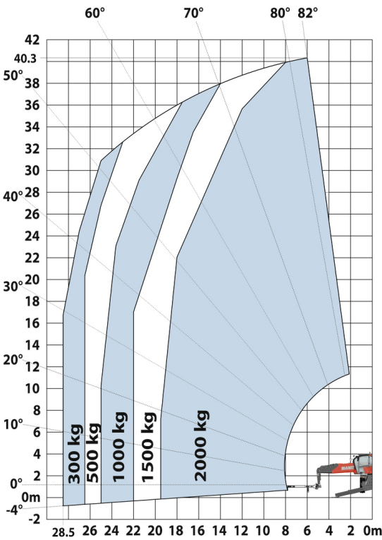
Drehung mit abgelassenen Stützen und 2 to jib (Metrisch) Maschine auf abgesenkten Stabilisatoren mit 1500 kg Winde (Metrisch)
