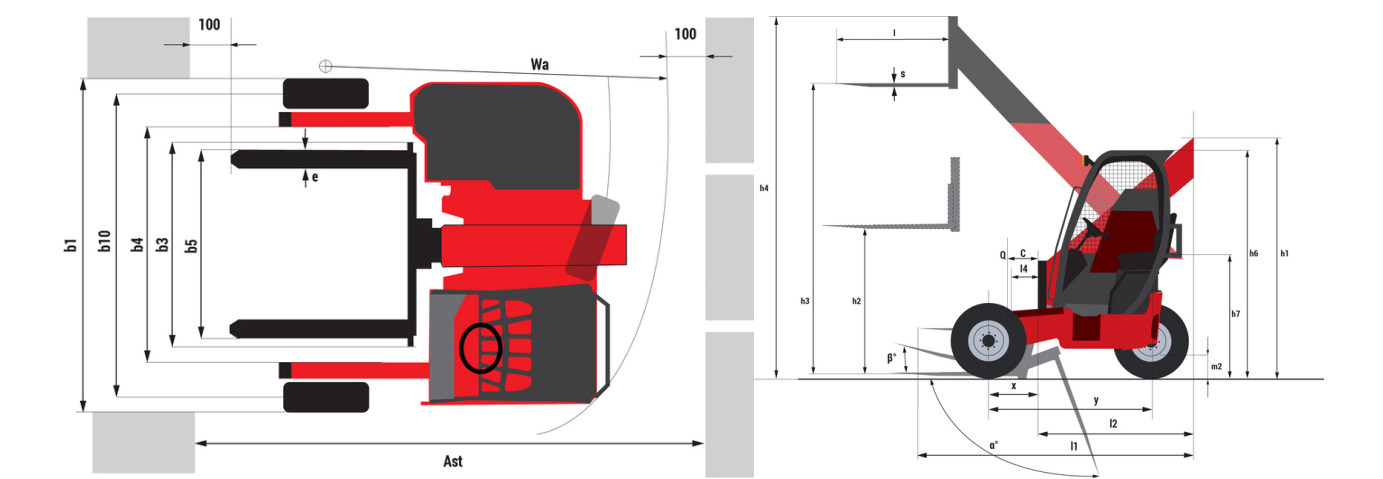
TMT 27P Y ST5 - Maßzeichnung
